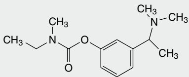
Rivastigmine
