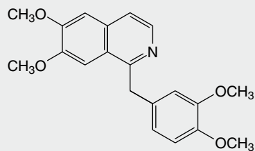
Papaverine
