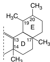
\alpha -Amyrin
