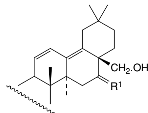
Saikosaponin b 2 , R^1 = \begin{matrix} \text{OH} \\ \diagup \\ \text{H} \end{matrix}
