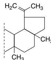
Lupeol
