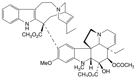
Vinorelbine
