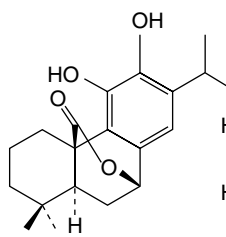
Carnosol
