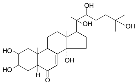
Ecdysterone
