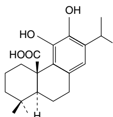
Carnosic acid
