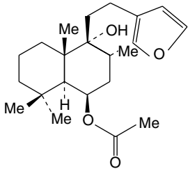
Rotundifuran (Labdane-type diterpenoid)
