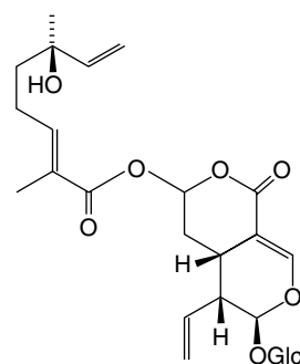
Menthiafolin
